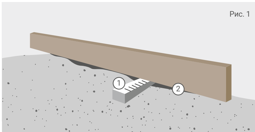
1 – Измерительный щуп. 2 – Отклонение поверхности слоя от плоскости.
